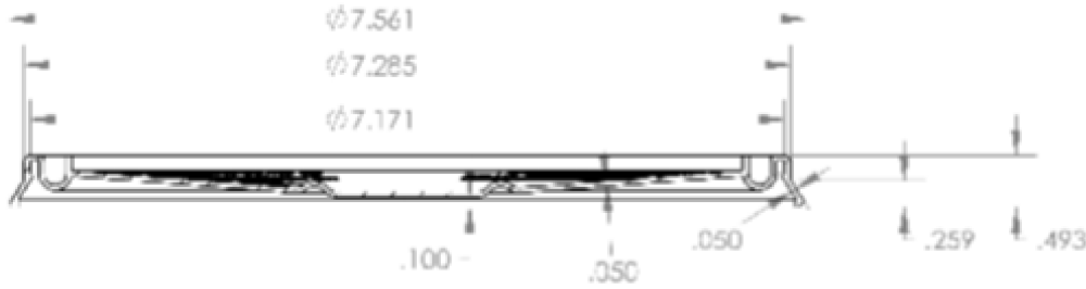
SECTION A-A SCALE 1 : 1.5
