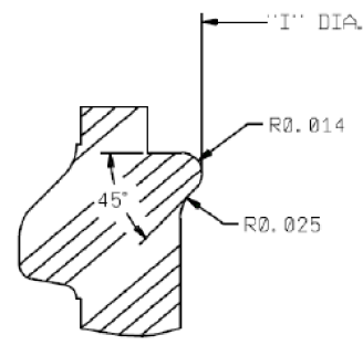
DETAIL "X" SCALE: 10 X 1
