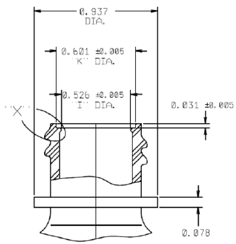
NECK DETAIL SCALE: 2 X 1
