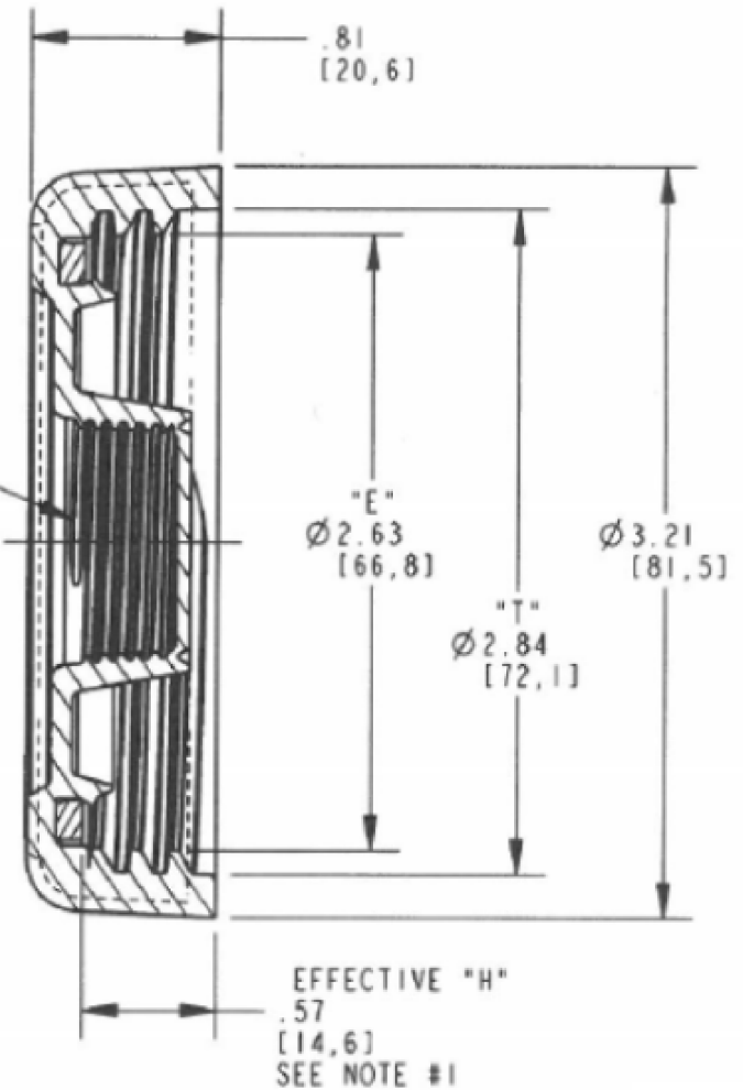
SECTION A-A
