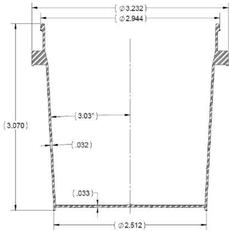
SECTION A-A SCALE 1.5 : 1
