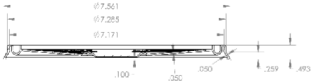
SECTION A-A SCALE 1 : 1.5
