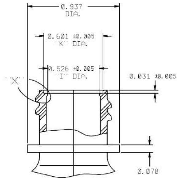
NECK DETAIL SCALE: 2 X 1
