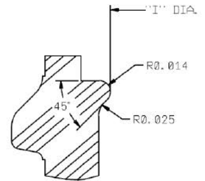
DETAIL "X" SCALE: 10 X 1
