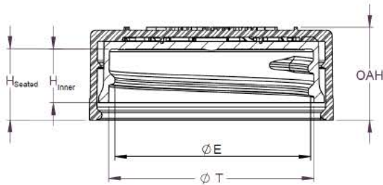
SECTION A-A SCALE 3 : 2
