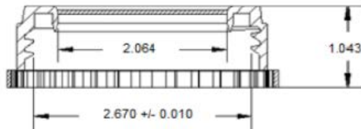
CAP DIMENSIONS
