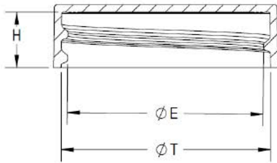
SECTION D-D
