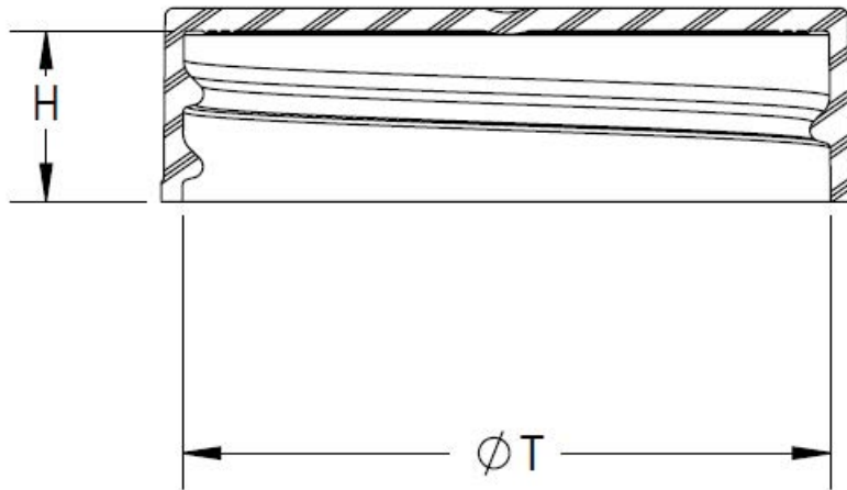
SECTION D-D
