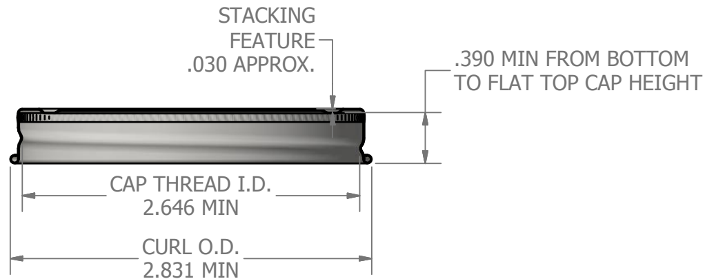
SECTION A-A SCALE 1 : 1
